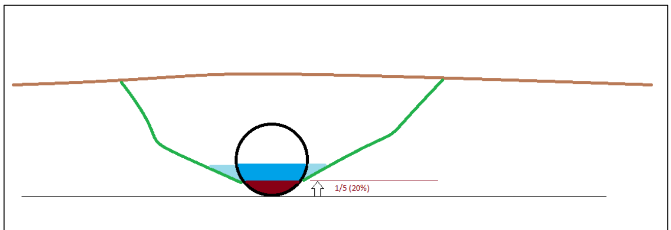
Figur 2. Principskitse for etablering af røroverkørsel.
